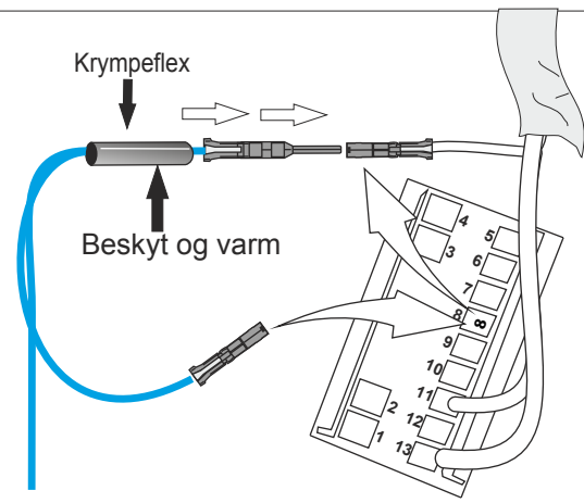
Afmonter ledning fra pin nr. 8 og indsæt blå fra DCS-CL-83
