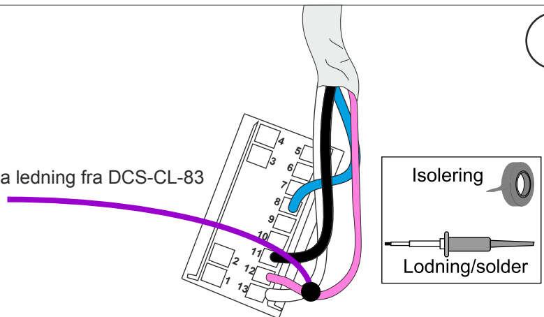
Lod lilla ledning fra DCS-CL-83 på ledningen i pin nr. 12.
