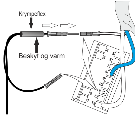
Afmonter ledning fra pin nr. 11 og indsæt sort fra DCS-CL-83
